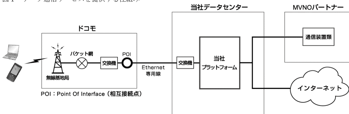
図1 データ通信サービスを提供する仕組み
